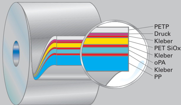
4-Schicht-Verbund
