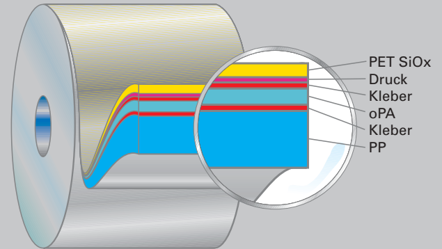
3-Schicht-Verbund
